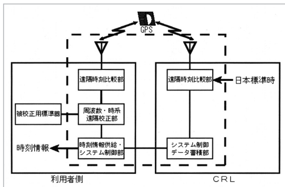
図4 遠隔校正システムの概要
