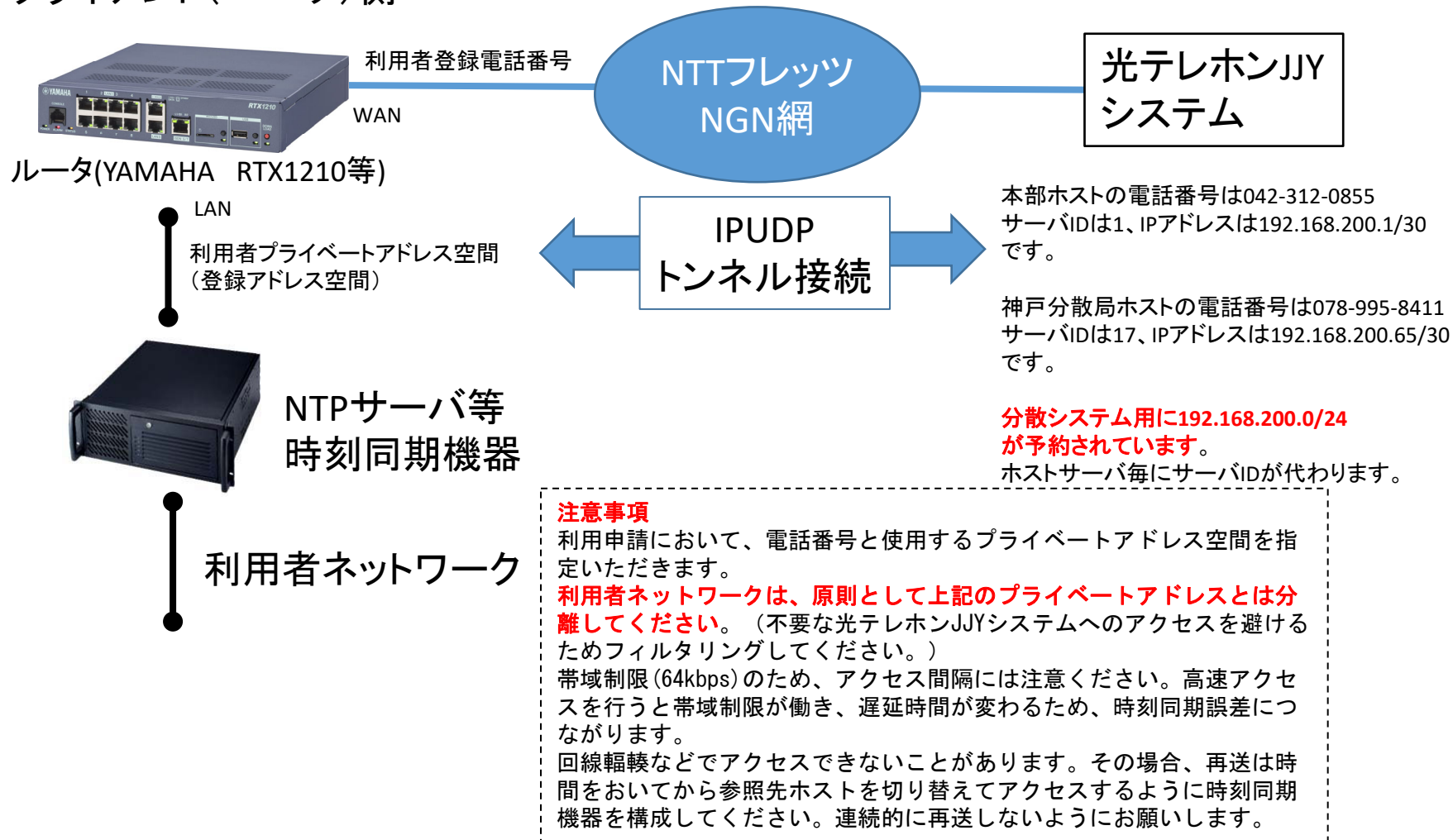
光テレホンJJY 利用接続図
